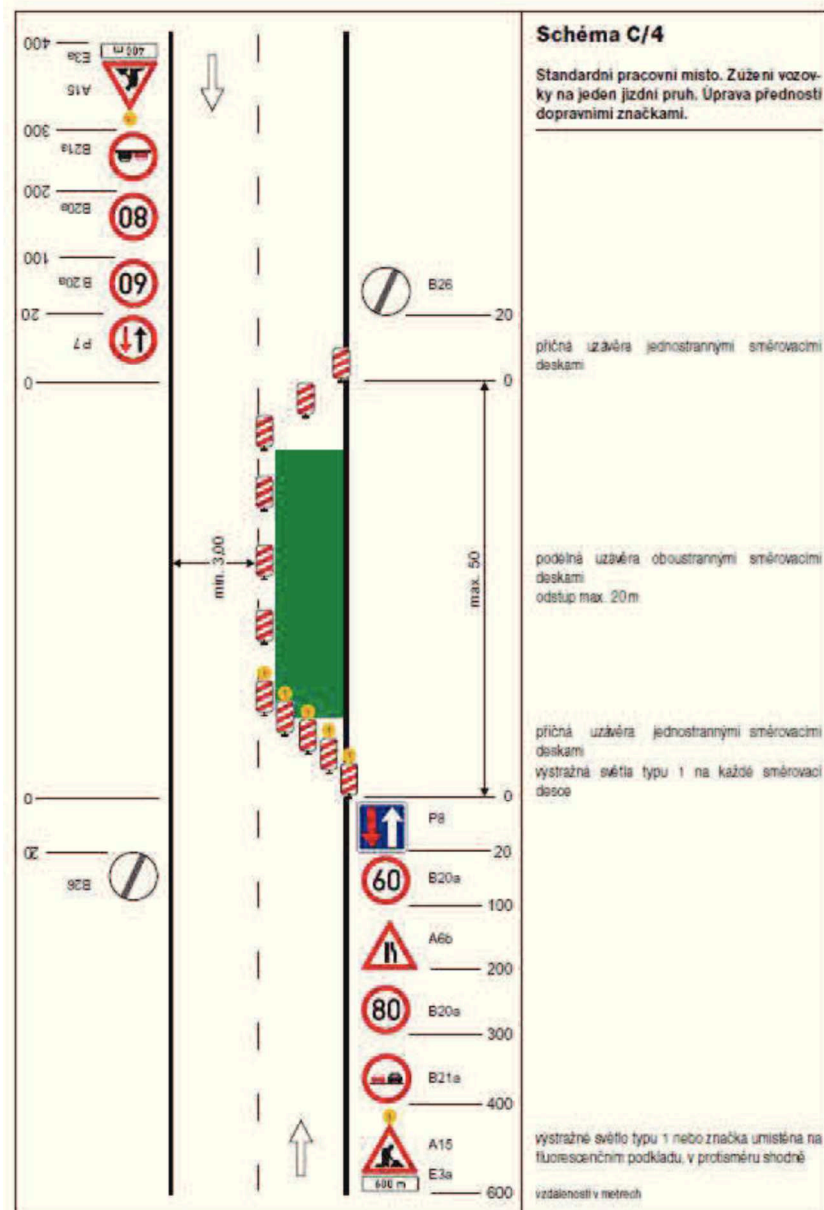
SCHEMATA PRO OZNAČENÍ PRACOVNÍCH MÍST MIMO OBEC
