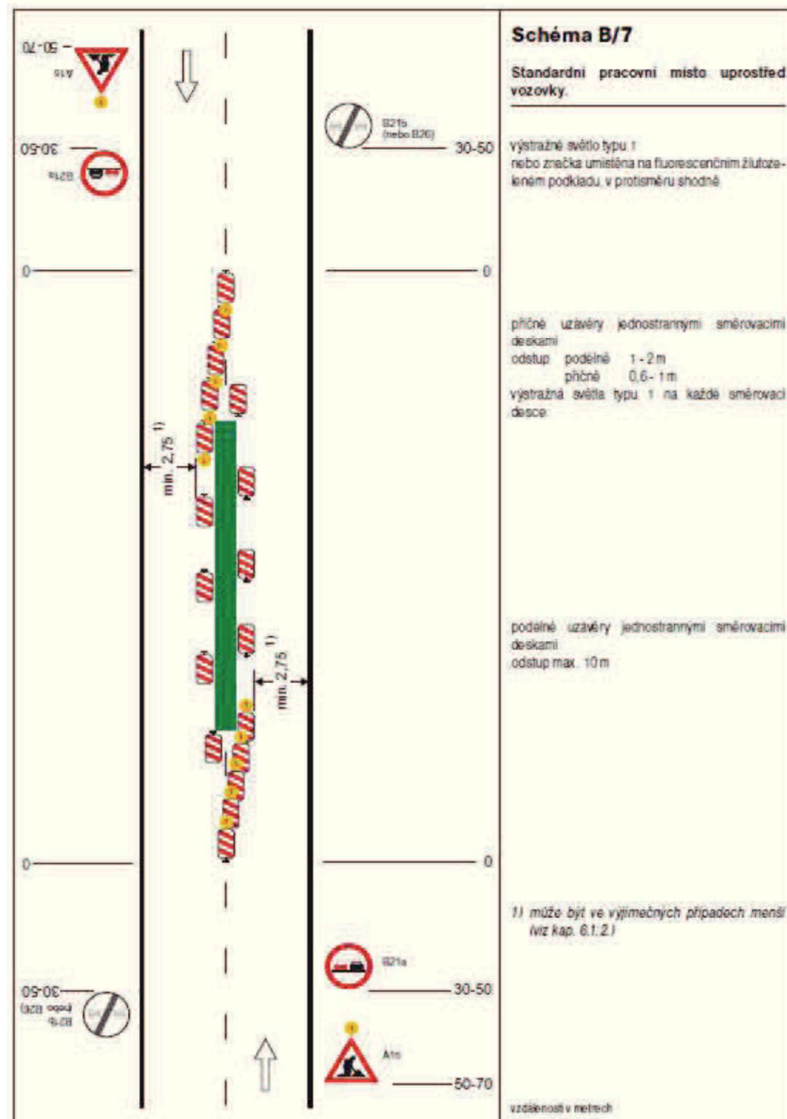
SCHEMATA PRO OZNAČENÍ PRACOVNÍCH MÍST V OBCI
