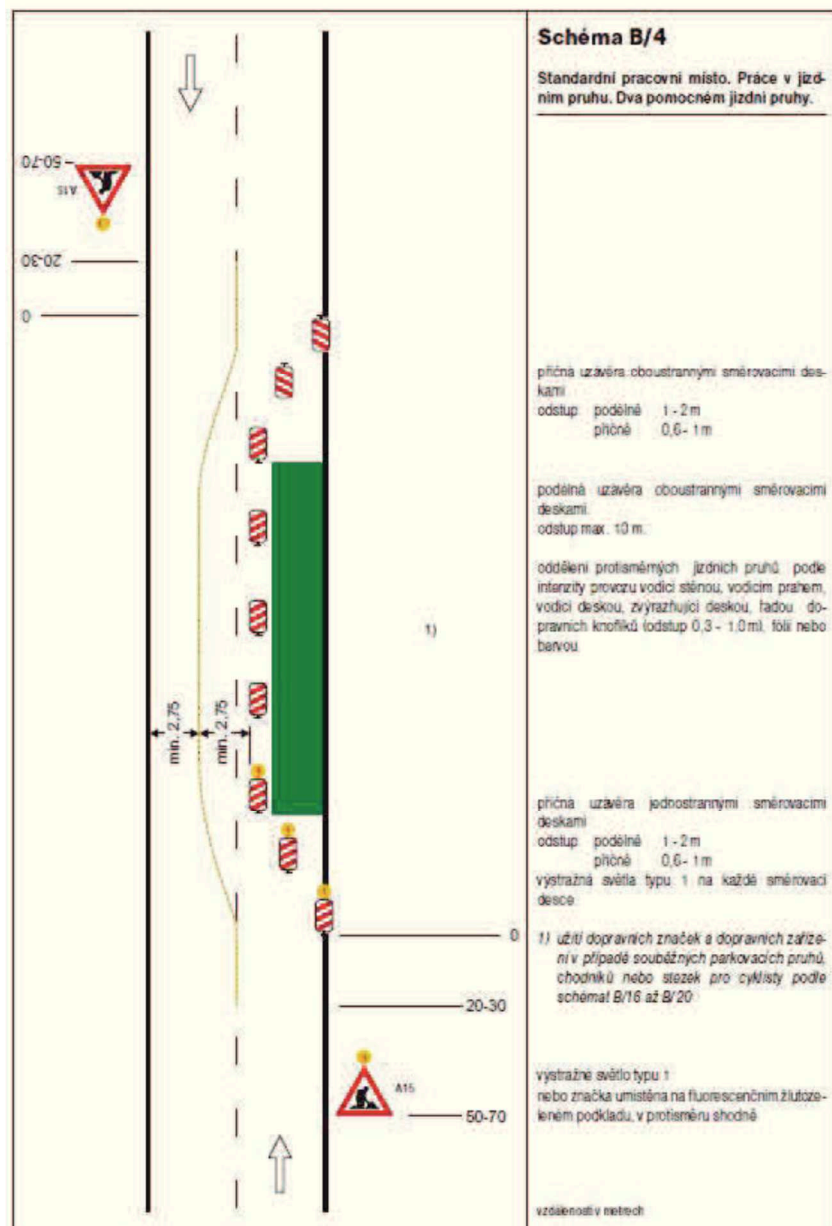
SCHEMATA PRO OZNACENÍ PRACOVNÍCH MÍST V OBCI
