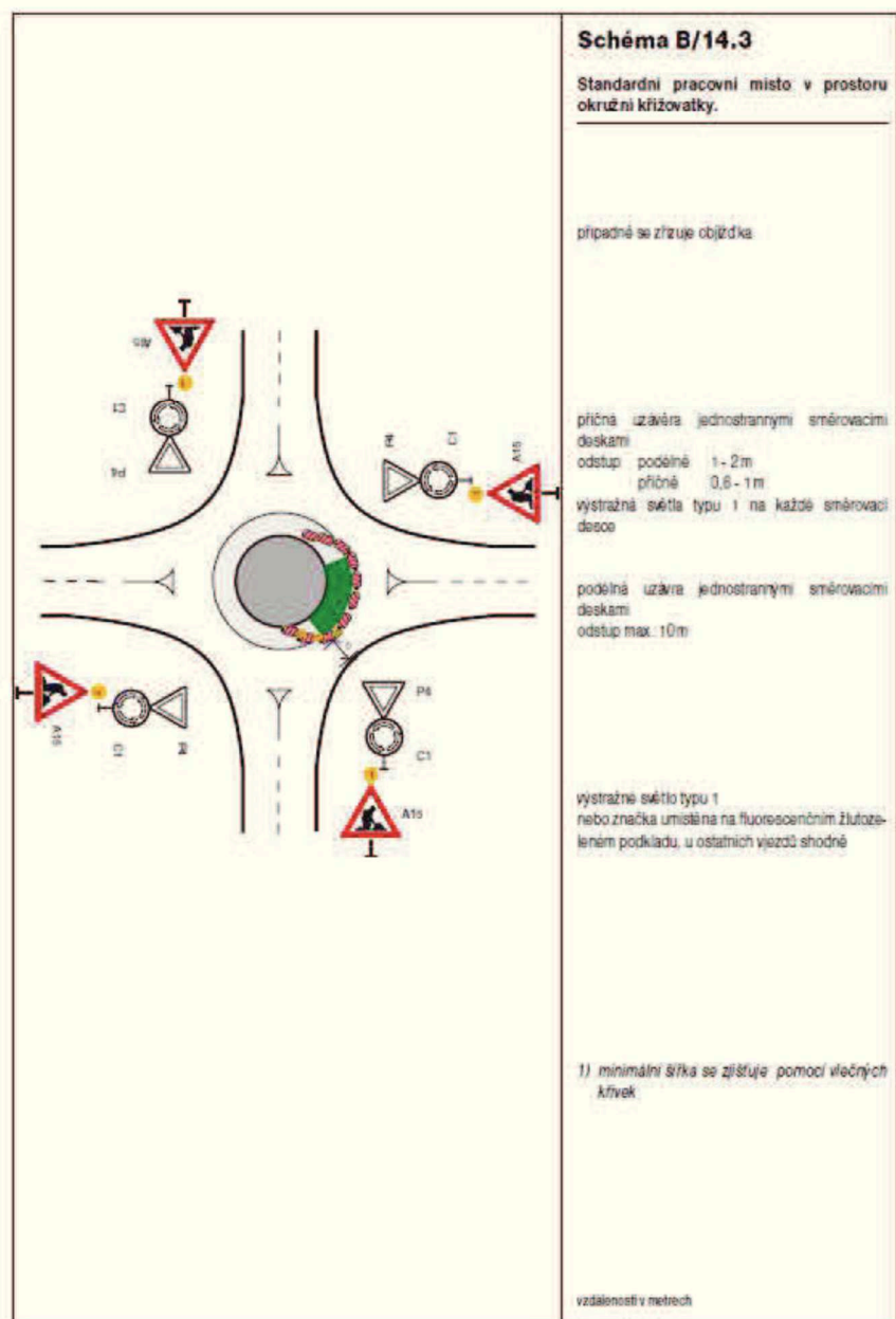
SCHEMATA PRO OZNAČENÍ PRACOVNÍCH MÍST V OBCI
