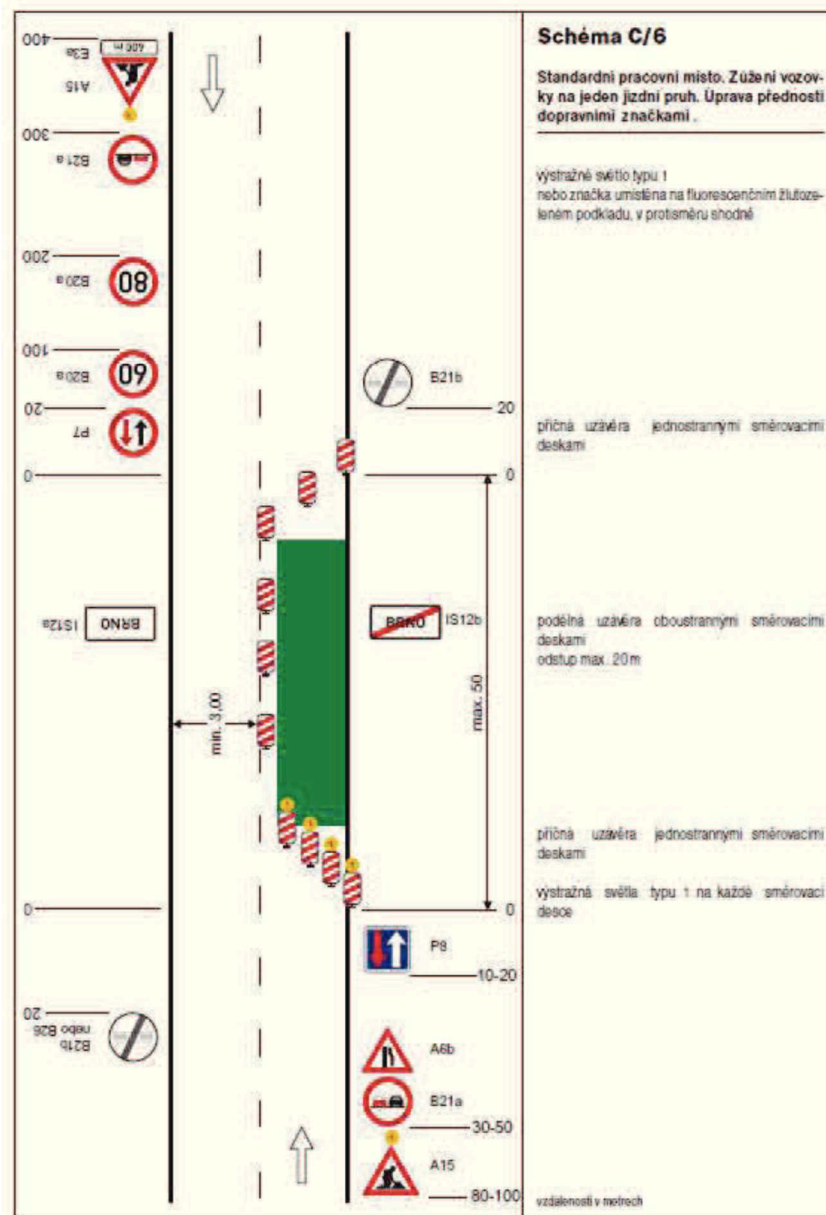
SCHEMATA PRO OZNAČENÍ PRACOVNÍCH MÍST MIMO OBEČ
