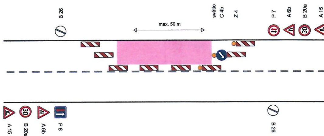
schéma 1
