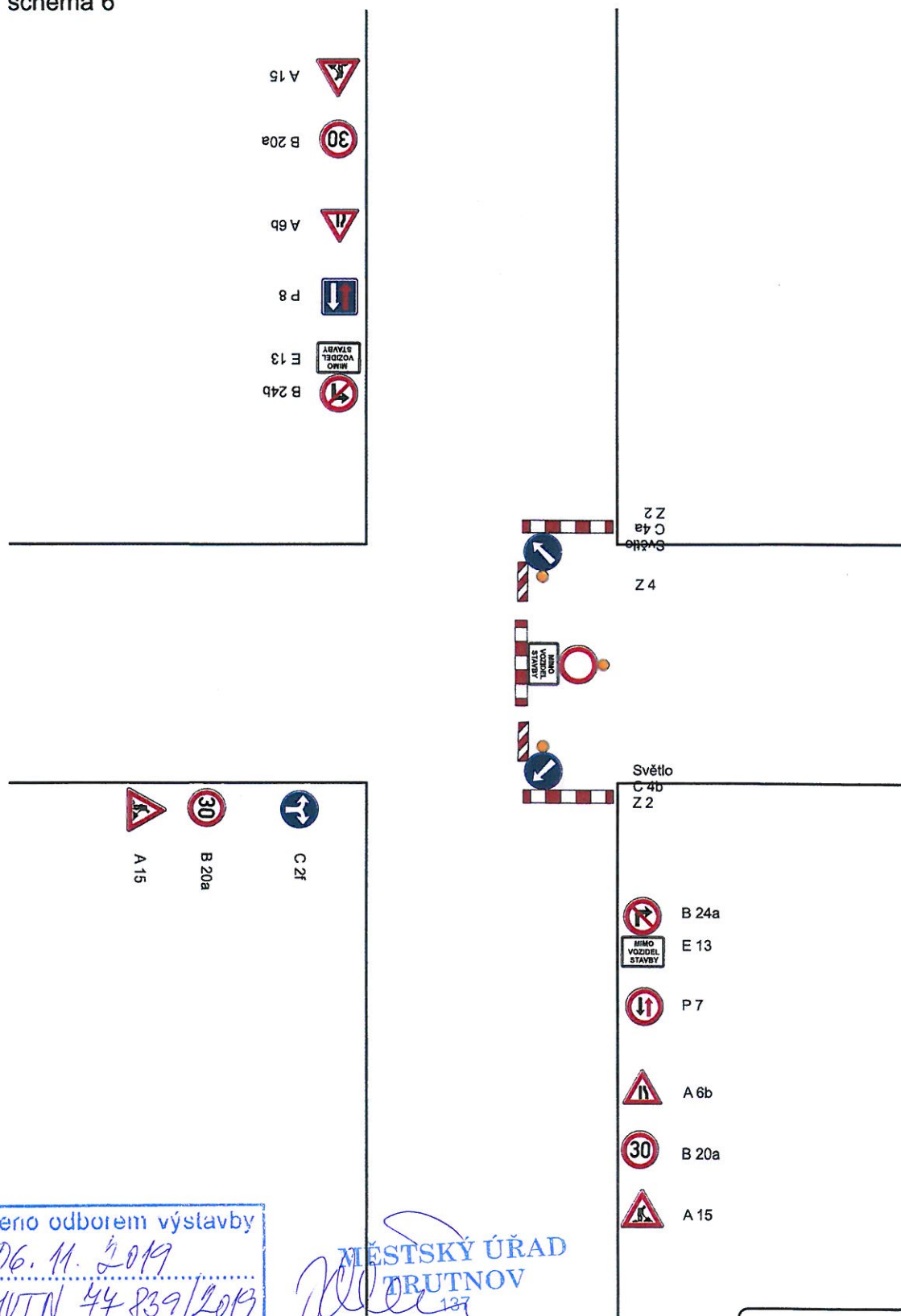
schéma 6
